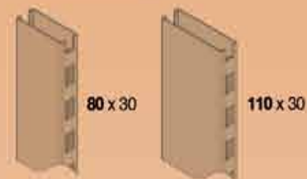
Montanti con asolatura passo 50 Pitch 50 slotted uprights
