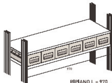
Cassettini larghezza mm. 320 in appoggio su ripiani Shelf-standing drawers L 320 mm
