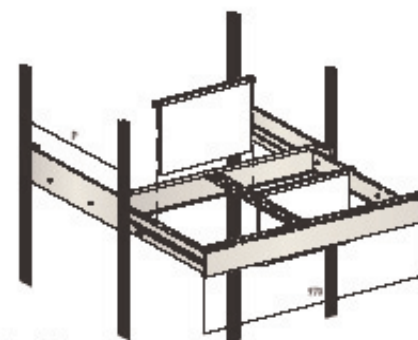
Telai estraibili per cartelle o tabulati sospesi Pull-out frame for suspension files
