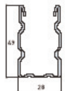
Sezione Cross-section
