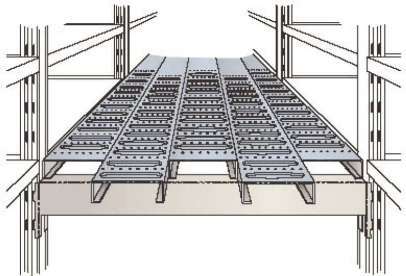
Ballatoio con piano di calpestio in pianetti di grigliato Platform with walkway in slatted sections
